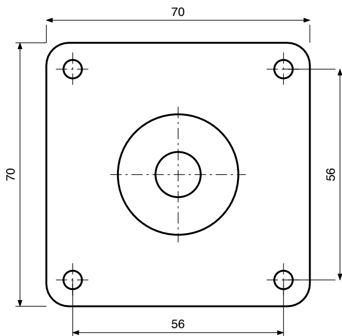
План · 4 отв. \varnothing 4.9 · отвір у випресовці \varnothing \sim 12
