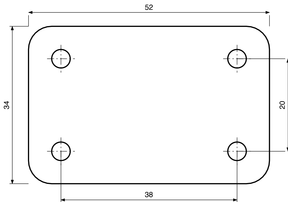
План · 4 отв. \varnothing 4
