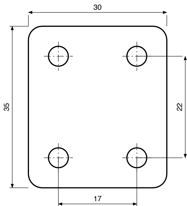
План · 4 отв. Ø4.3
