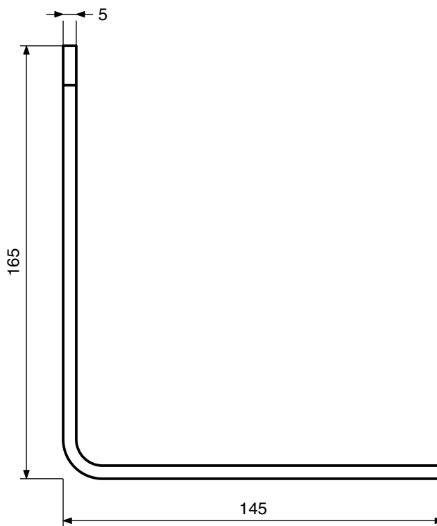
Вид збоку
