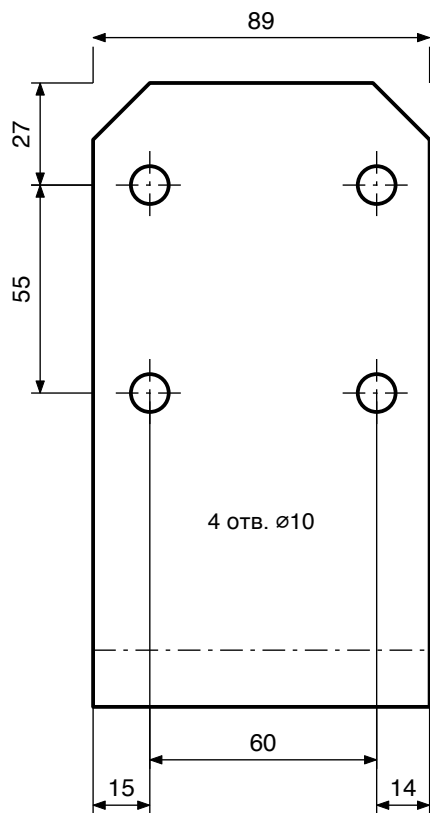
Вид спереду
