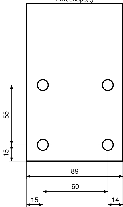
Вид знизу · 4 отв. \varnothing 10
