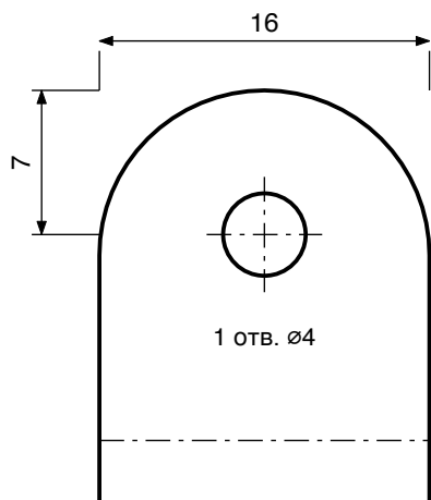
Вид спереду
