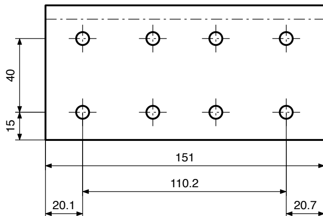
Вид знизу · 8 отв. \varnothing 7
