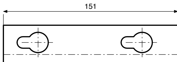
Вид спереду · 2 пази \varnothing 17.7
