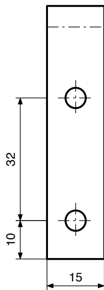
Вид знизу · 2 отв. \varnothing 5.3
