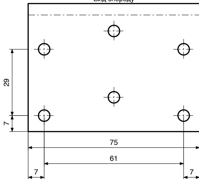
Вид снизу · 6 отв. \varnothing 5
