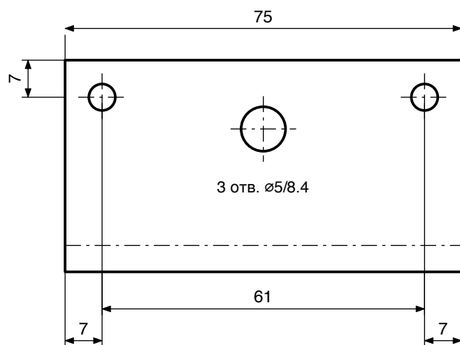
Вид спереду
