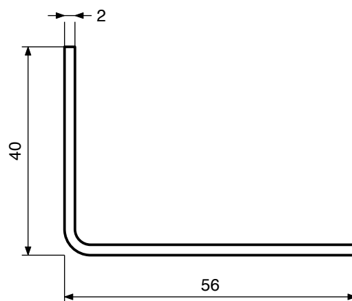
Вид збоку
