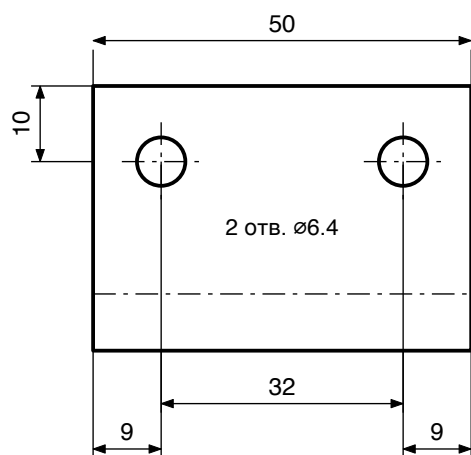
Вид спереду
