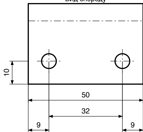
Вид снизу · 2 отв. Ø6.4
