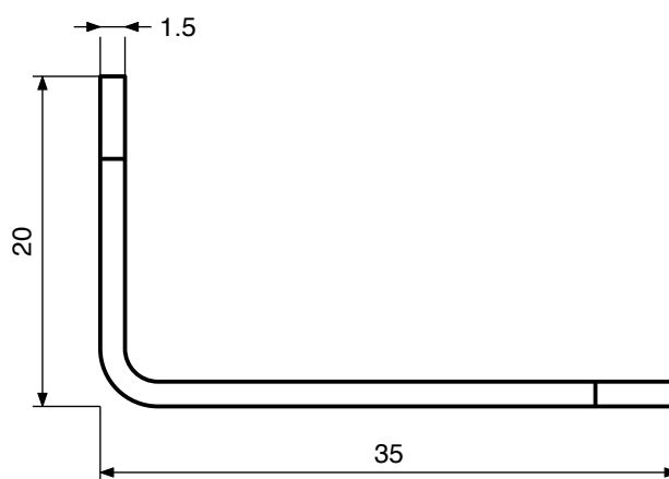
Вид збоку
