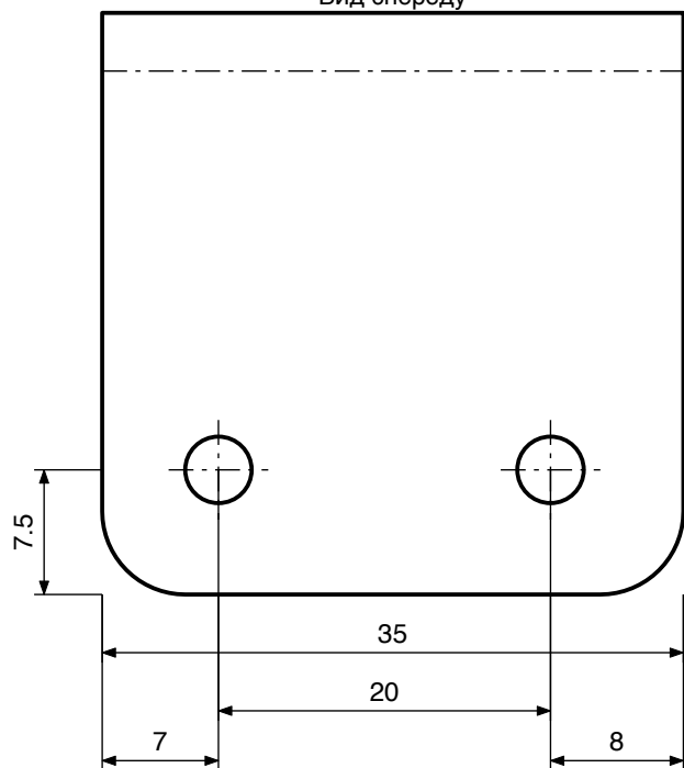
Вид снизу · 2 отв. Ø4
