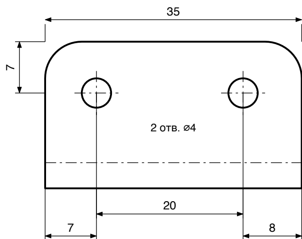
Вид спереду
