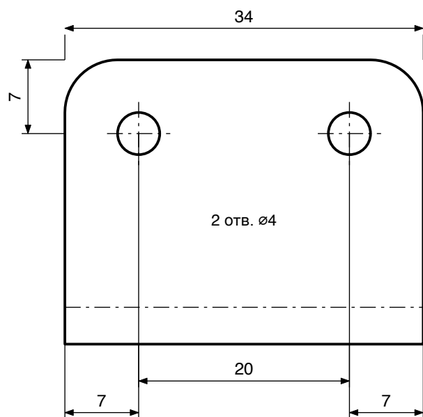
Вид спереду
