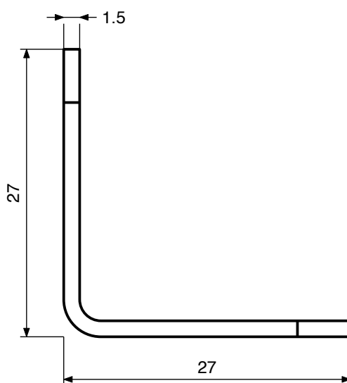
Вид збоку
