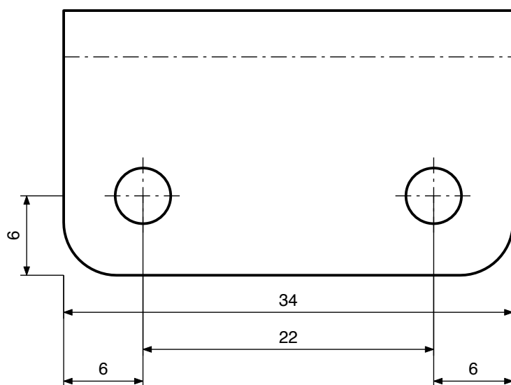
Вид знизу · 2 отв. Ø4.2
