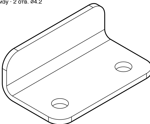
Ізометрія
