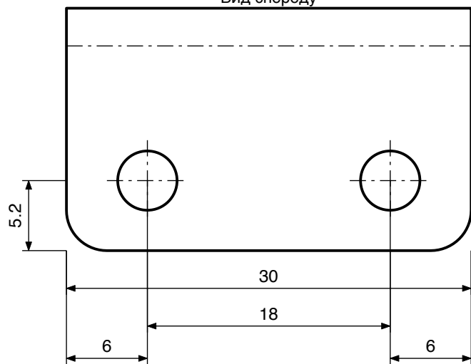
Вид спереду
