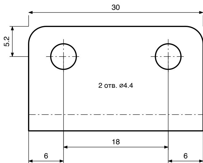
Вид спереду
